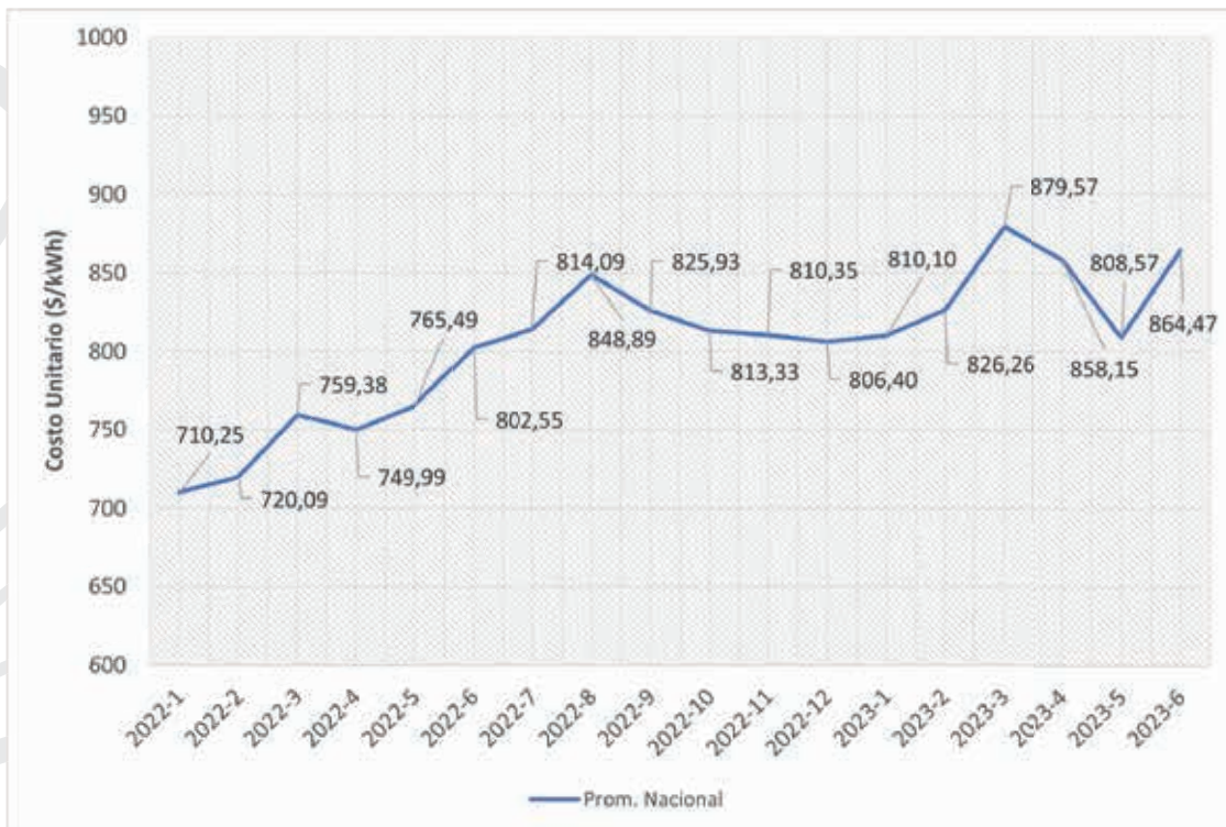
Figura 2.6 Comportamiento del CU, promedio nacional
